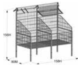
PSM007 UPPSTÄLLNING – TRADITIONELL BORD 80X160
