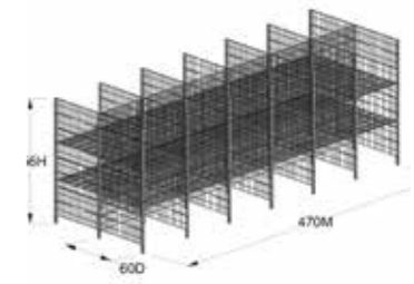
PSM081 UPPSTÄLLNING – 120X160
