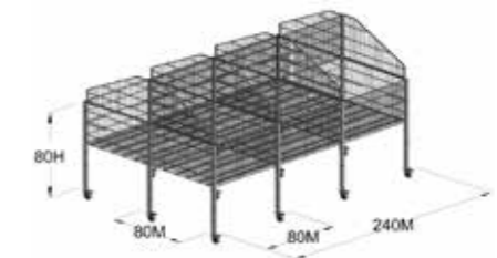
PSM078 UPPSTÄLLNING – BORD 80 X 240 MED 6 FACK
