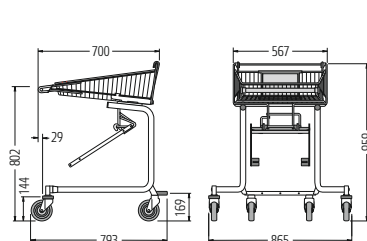
EKW FÜR ROLLSTUHLFAHRER 40
