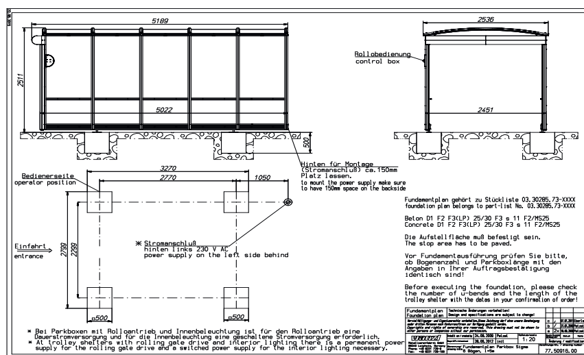
Beispiel eines Fundamentplans
