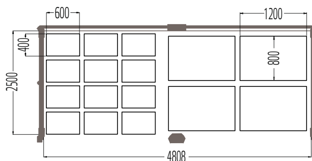
Plano de ejemplo para un llenado práctico con palés (vista de planta)
