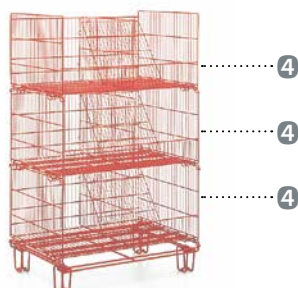
STP/R 810 con rivestimento colorato (a richiesta), con telaio inferiore fisso, griglie di separazione, ripiani inclinati
