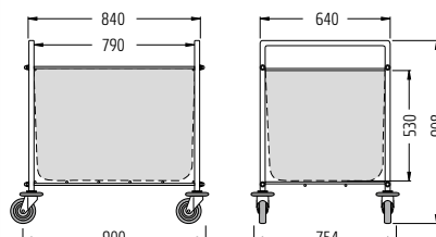
Chariot de collecte LT 240
