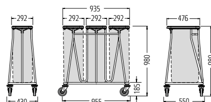
SW 1/80
