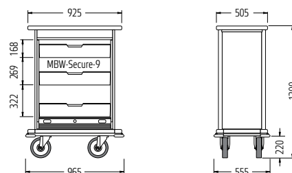
Dostępne również inne wymiary modelu MBW-Smart – zgodnie ze stroną 5.
