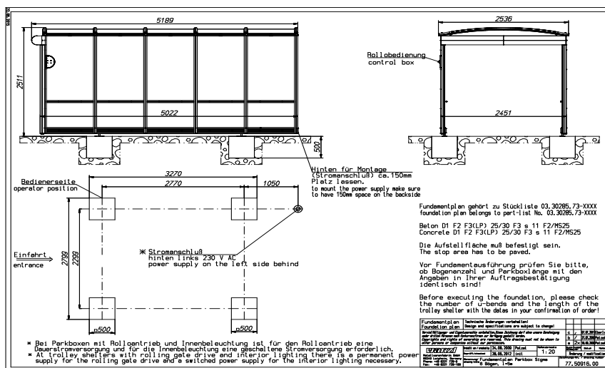
Exemple d'un plan des fondations
