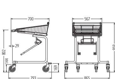
CHARIOT LIBRE-SERVICE POUR PER-SONNES EN FAUTEUIL ROULANT 40
