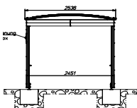
05 FONDATIONS D'ABRIS POUR CHARIOTS
