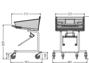
CHARIOT LIBRE-SERVICE POUR PER-SONNES EN FAUTEUIL ROULANT 90
