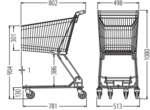
D 90 RC
