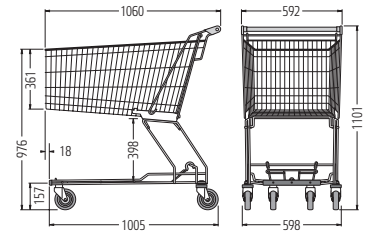
D 185 RC
