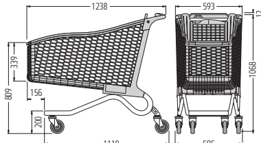
TANGO 240 E
