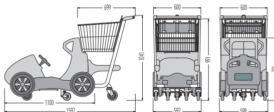
FUN CABRIO 80
