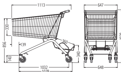
ELX 248 B
