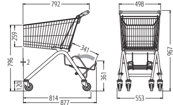
ELX 75
