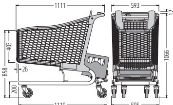
TANGO 220 P
