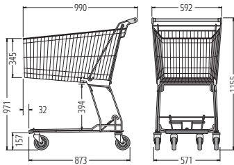
D 150 RC
