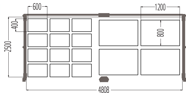
Plano de ejemplo para un llenado práctico con palés (vista de planta)
