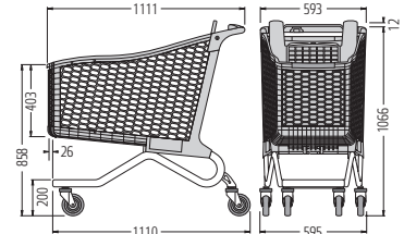
TANGO 220 E
