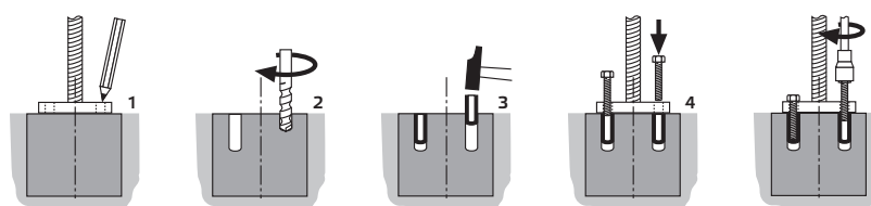
Colocar el refugio para carros, trazar el punto de perforación / Perforar los orificios para los tacos, Ø 14 mm / Insertar los tacos a ras / Colocar el refugio para carros en posición, introducir los tornillos de fijación / Apretar los tornillos de fijación
