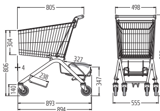
ELX 90
