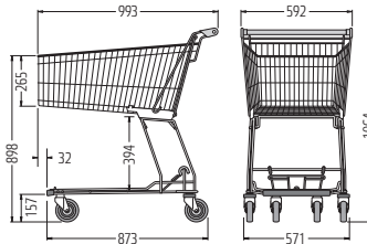
D 120 RC
