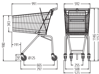
ELT 7/150
