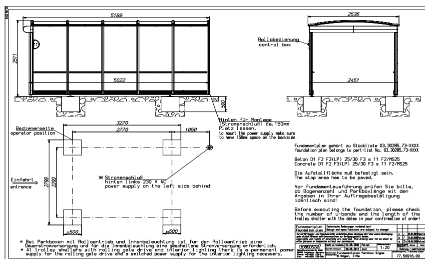
Ejemplo de plano de cimientos
