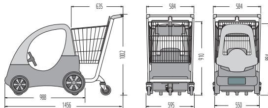
FUN MOBIL 80
