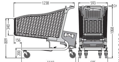
TANGO 240 P
