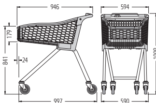
TANGO 90 E
