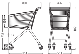
EL 90
