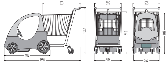
FUN MOBIL 130
