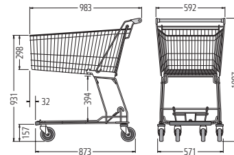
D 130 RC
