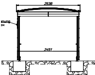
05 CIMIENTOS PARA REFUGIOS PARA CARROS
