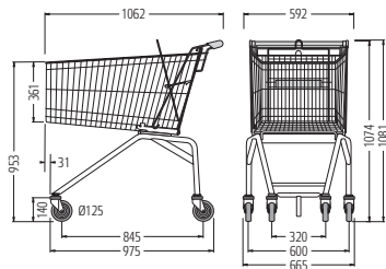
ELT 9F/185*
