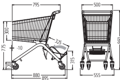
02 DIMENSIONES DE LOS CARROS DE AUTOSERVICIO
