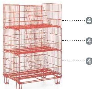
STP/R 810 revêtement coloré (sur demande), avec châssis fixe, grilles de séparation, grilles en biseau
