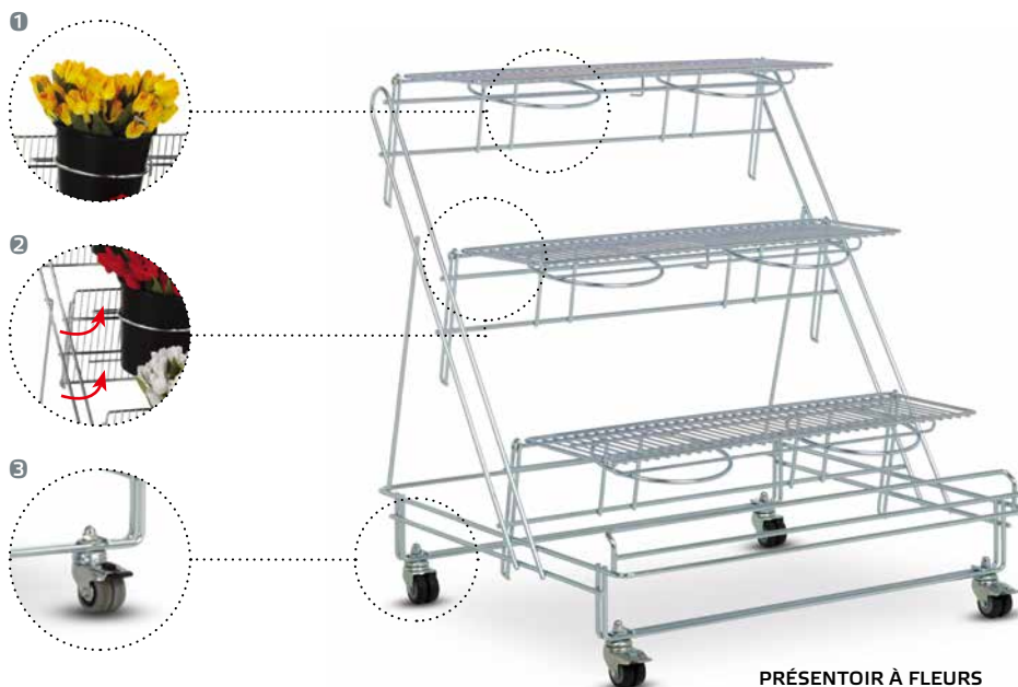
PRÉSENTOIR À FLEURS VARIO avec six porte-seaux, tablette fil repliée
