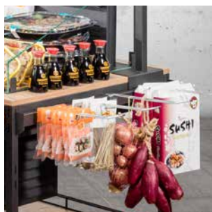
Rail support avec crochets doubles
