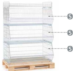
3 STP 812 avec panier supérieur, installé sur une palette
