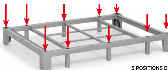
5 POSITIONS DE MONTAGE des parois latérales pour une infinité de constructions.
