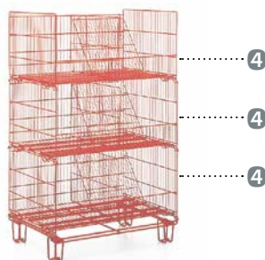
STP/R 810 con revestimiento de color (por encargo), con chasis fijo, separadores de varilla, emparrillados inclinados
