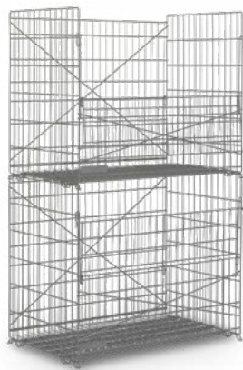
↑ STAPELBARE LAGERKÖRBE mit abklappbarem Frontgitter
