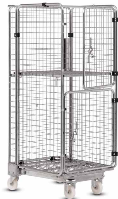
RC/N2 Modelo básico con estante de varilla abatible (de serie)
