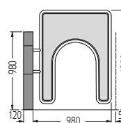
AUTOMATIC ACCESS DOOR Child passage door
